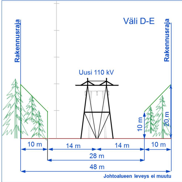
Kuva 1-5. Poikkileikkauskuvaa uuden voimajohdon sijoittumisesta olemassa olevaan voimajohtoalueeseen välillä D-E ja valokuva nykyisestä voimajohdosta.
