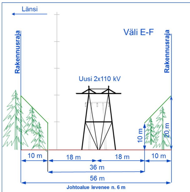
Kuva 1-6. Poikkileikkauskuvaa uuden voimajohdon sijoittumisesta olemassa olevaan voimajohtoalueeseen välillä E-F ja valokuva nykyisestä voimajohdosta.
