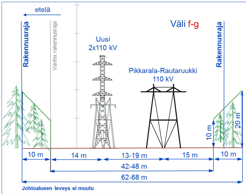
Kuva 1-8. Poikkileikkauskuva uuden voimajohdon sijoittumisesta yhteispylväisiin olemassa olevan voimajohtoreitin yhteyteen välillä f-g.
